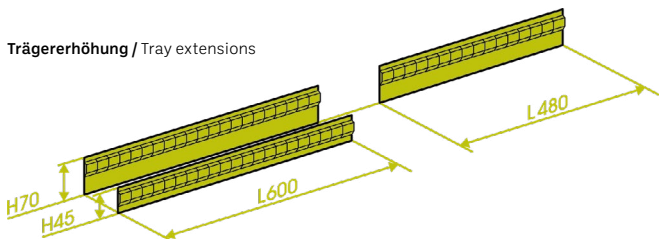
Trägererhöhung / Tray extensions
